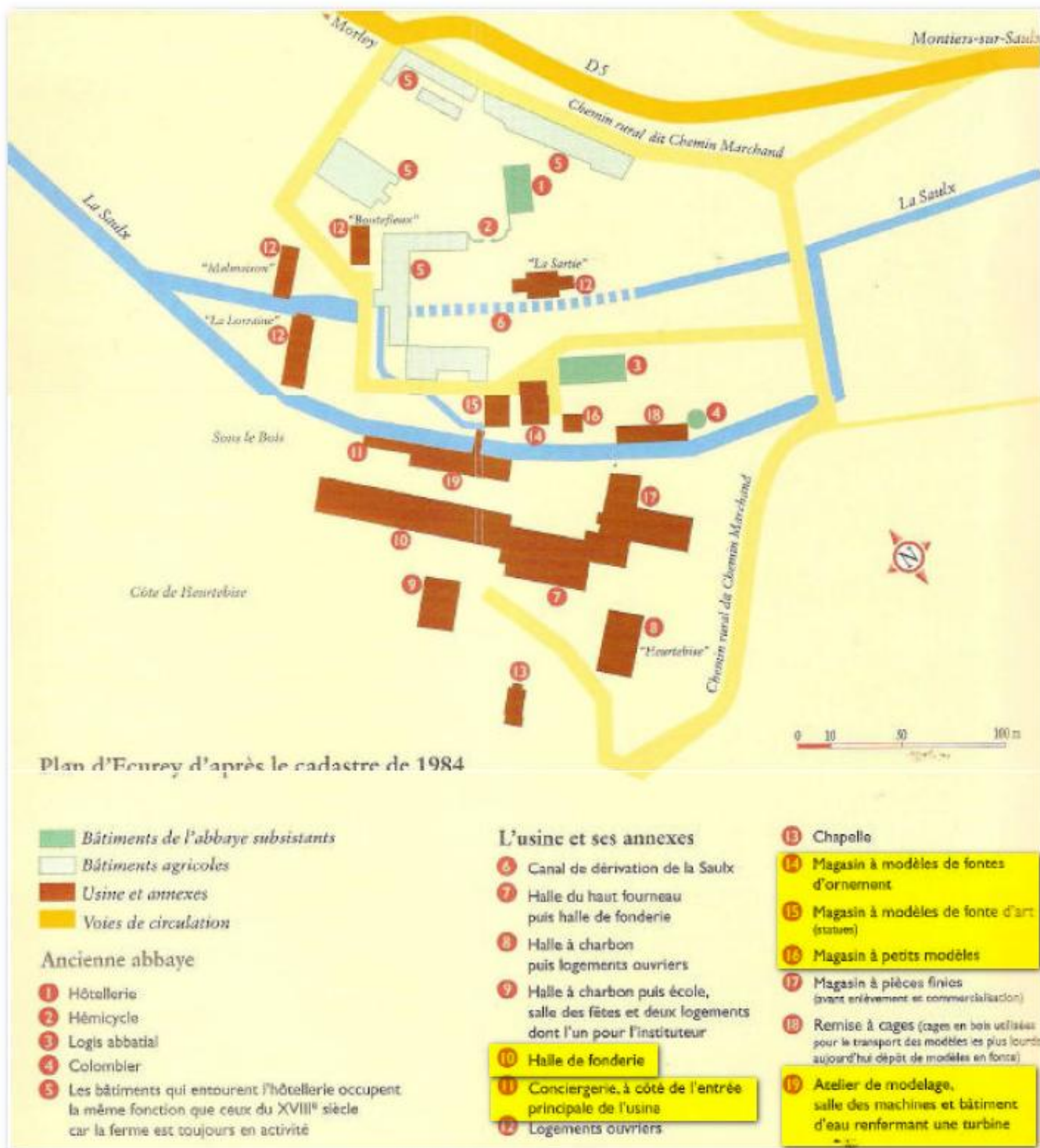
Plan du site des Fonderies d'Écurey
